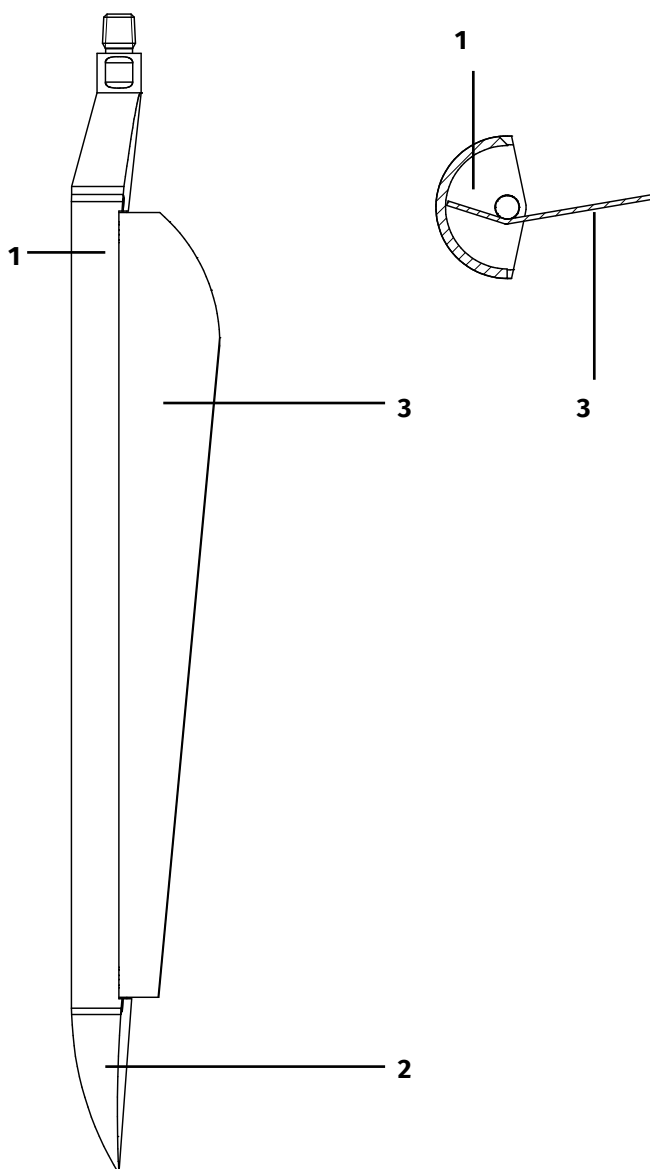
Veenboor, zijaanzicht (links) en dwarsdoorsnede (rechts).
